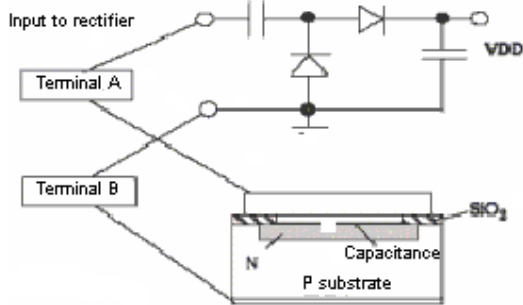
Fig. 3.6.3 μ-chip rectifier 38
